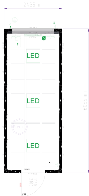
20ft Raum-Modul p0100581-004
