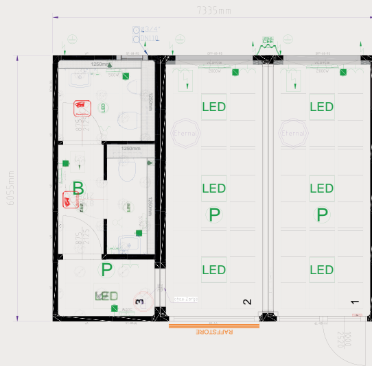
3er Premium-Anlage (3 x 20ft) mit Damen/Herren-WC p0101928
