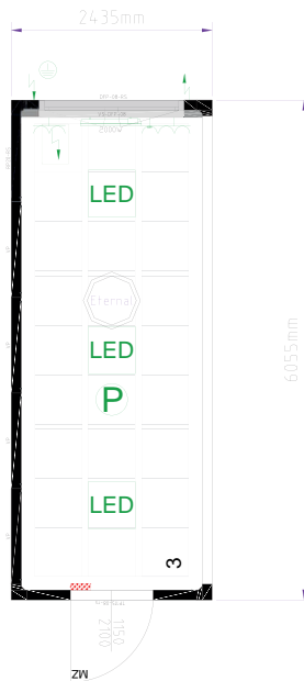
20ft Halbschale links mit Tür p0400062
