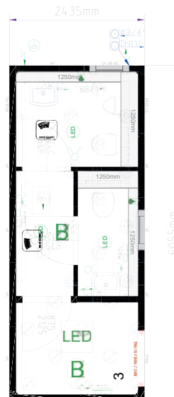
20ft Sanitär-Modul: Damen/ Herren-WC mit Zugang links p0101075-004
