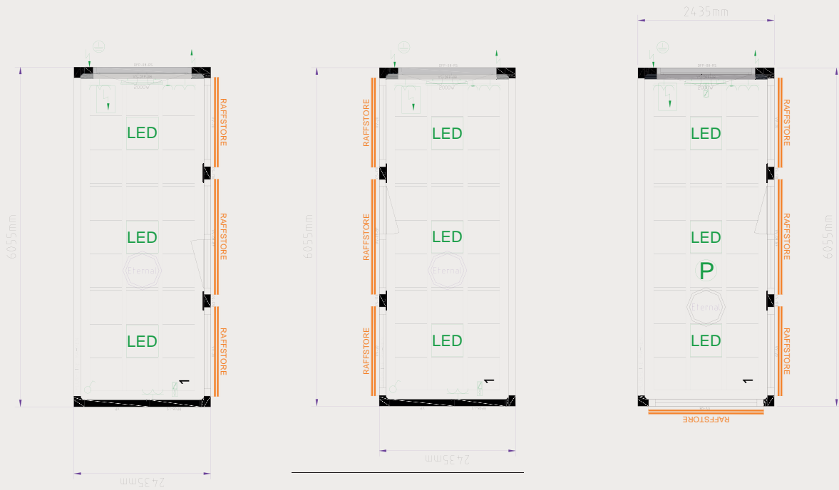
20ft Halbschale rechts mit Fenster/Raffstore p0100074-002
