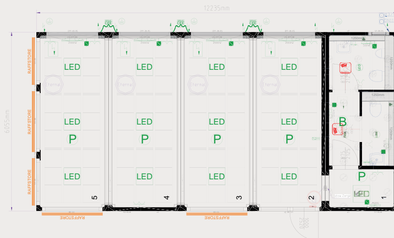
5er Premium-Anlage (5 x 20ft) mit Damen/Herren-WC und große Glasfronten mit Raffstores p0101924
