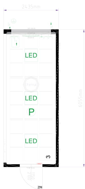
20ft Halbschale rechts mit Tür p0400062-004
